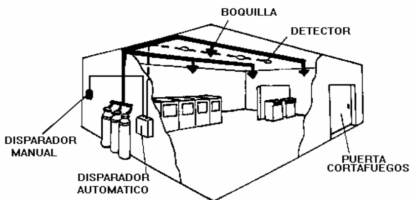
SISTEMA FIJO DE HALON DE APLICACION LOCAL
