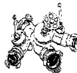
GEMELO DIVERGENTE VARIEDAD "TRIFURCACION"
