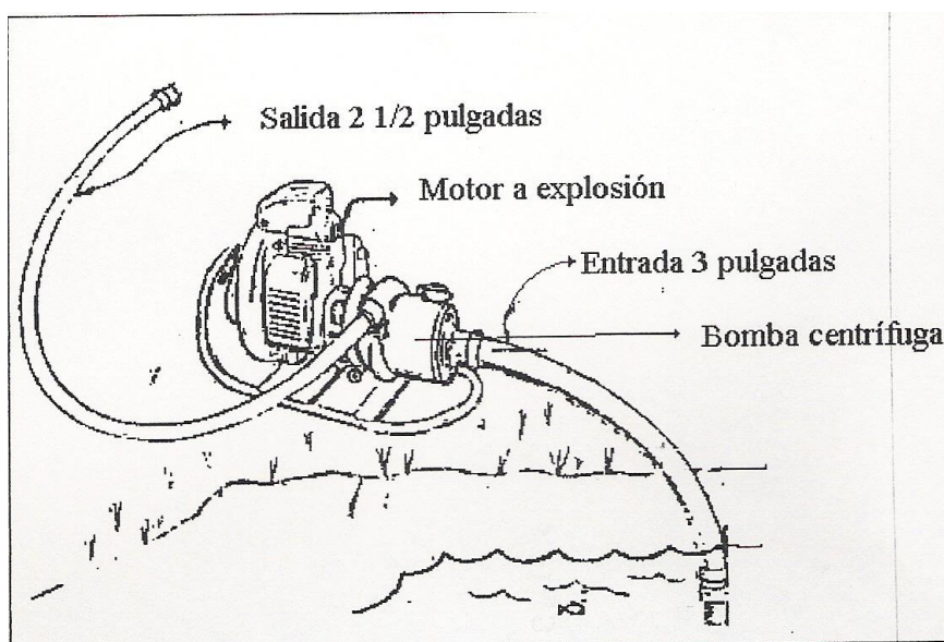
Esquema tipo de instalación de una motobomba portátil.
